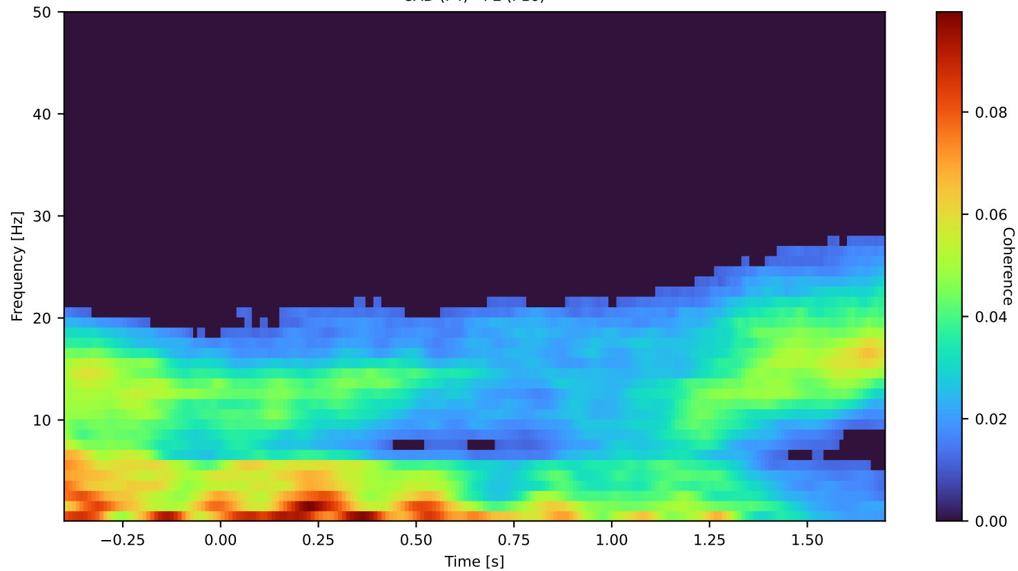
8AD (F4) - PE (P16)
